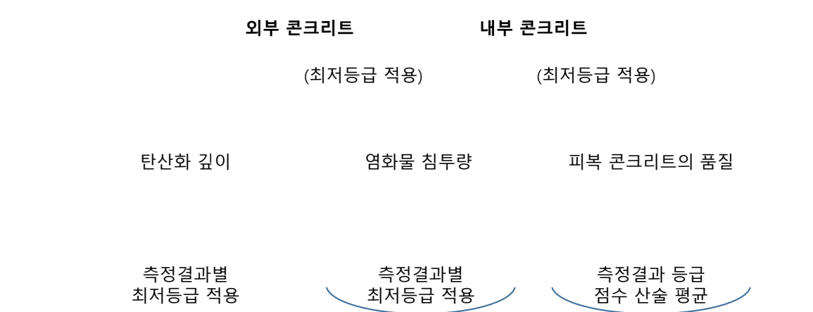
[그림 5.2] 콘크리트 내구성능 항목별 세부 평가방법
